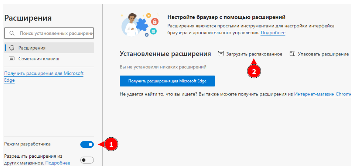
Рисунок 10-16. Загрузка распакованного расширения
