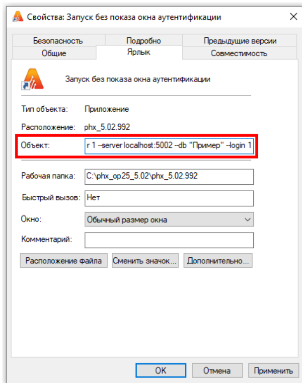
Рисунок 12-7. Добавление параметров командной строки в ярлык приложения (клиент версии 5.x)
