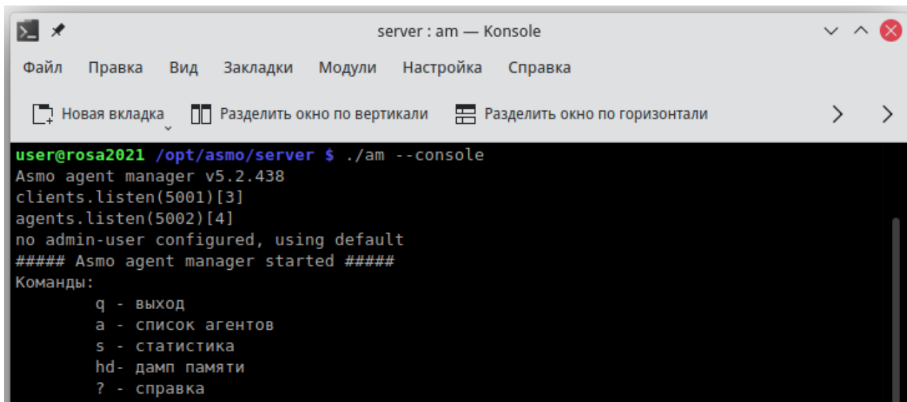
Рисунок 6-2. Проверка работоспособности менеджера агентов
