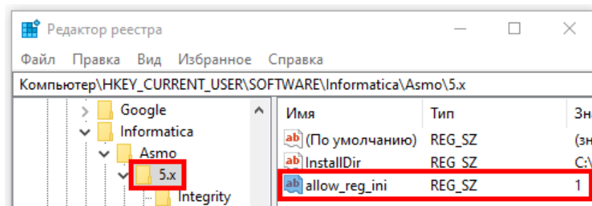
Рисунок 12-10. Окно редактора реестра с установленным параметром allow_reg_ini
