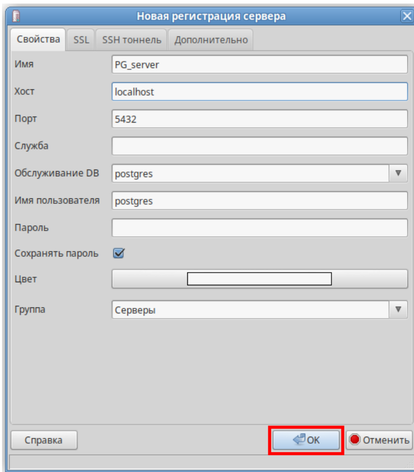
Рисунок 8-21. Регистрация нового сервера PostgreSQL
