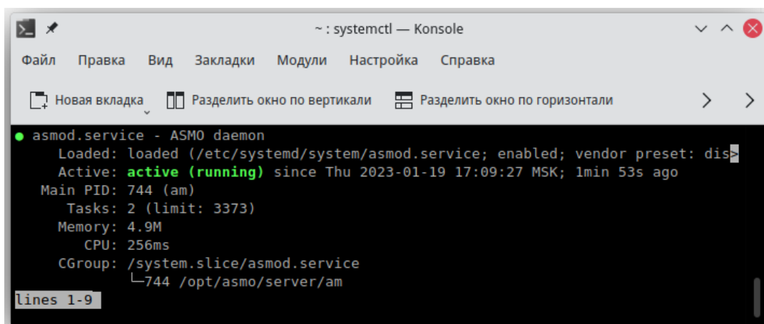
Рисунок 6-3. Проверка работоспособности службы asmod
