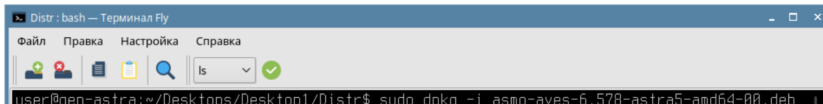
Рисунок 4-10. Ввод команды для установки через терминал
