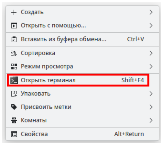
Рисунок 5-2. Запуск терминала
