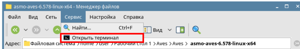
Рисунок 4-3. Запуск терминала
