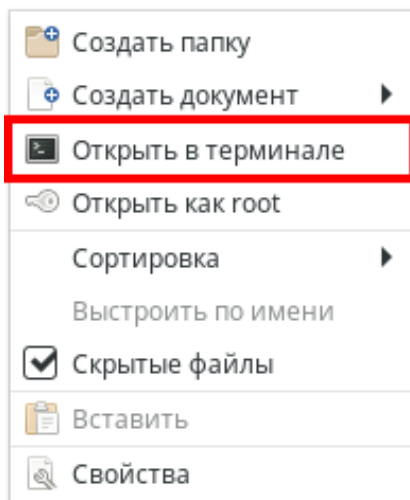
Рисунок 7-6. Запуск терминала
