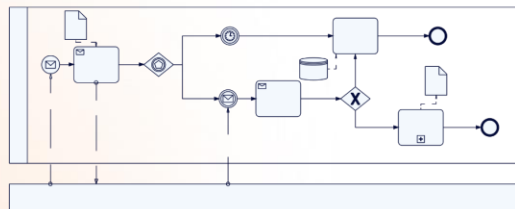
Схемы BPMN
