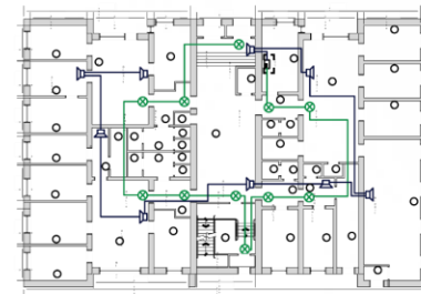
Планы этажей
