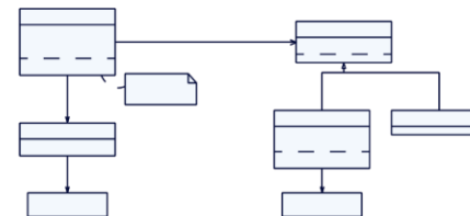
Диаграммы классов
